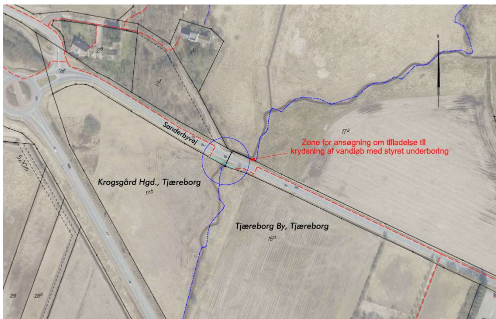
Figur 1: Fiberkablets krydsning af Krogsgård Møllebæk i st. 1632 m. Den rødstiplede linje viser det projekterede tracé for fiberkablet, mens den lyseblå linje viser tracéet for den styrede underboring af vandløbet.
